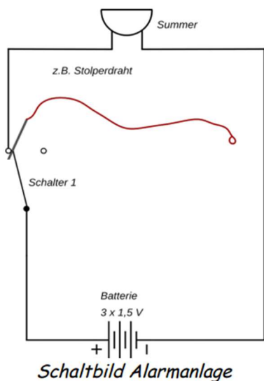
Šema sklopa alarmnog sustava/sistema
